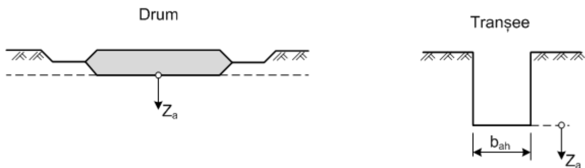
Figura Recomandări și cerințe minimale privind dispunerea în plan și adâncimea forajelor geotehnice.6: Drumuri și piste pentru aeroporturi
