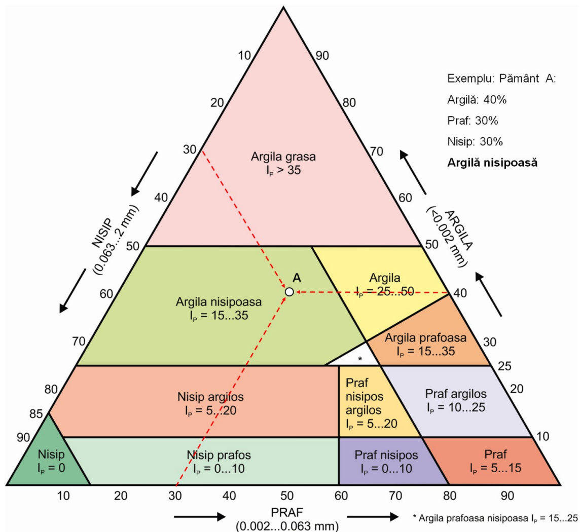
Figura O clasificare a pământurilor din punct de vedere granulometric.10: Diagrama ternară
