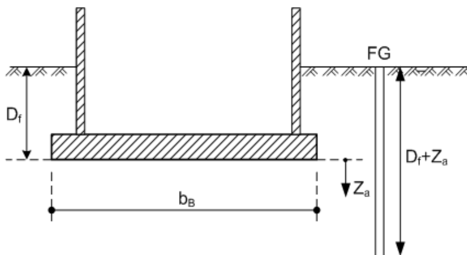
Figura Recomandări și cerințe minimale privind dispunerea în plan și adâncimea forajelor geotehnice.3: Fundații tip radier general
