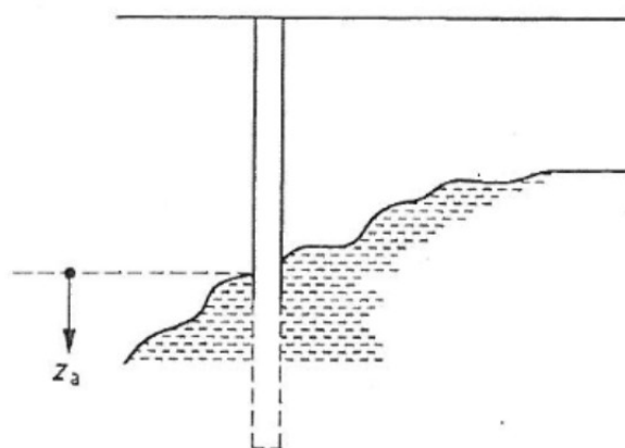
Figura Recomandări și cerințe minimale privind dispunerea în plan și adâncimea forajelor geotehnice.9: Perete de etanșare
