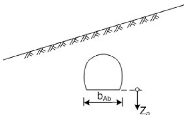
Figura Recomandări și cerințe minimale privind dispunerea în plan și adâncimea forajelor geotehnice.7: Tuneluri și excavații subterane
