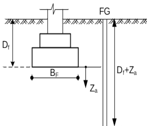
Figura Recomandări și cerințe minimale privind dispunerea în plan și adâncimea forajelor geotehnice.2: Fundații izolate sau continue
